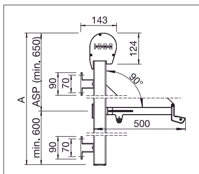
Cofre redondo a la vista
