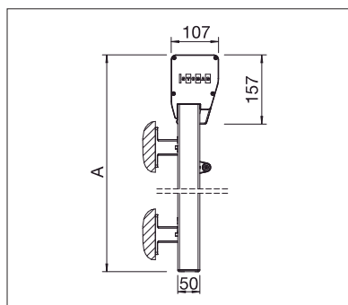
Cofre cuadrado retraído
