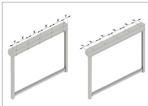
recomendaciones para fijación a pared y a techo
