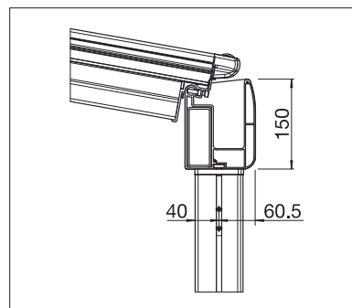
GP5100 | GP5110 Canal integrado desagüe
