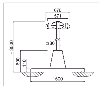
Base de hormigón y toldo vertical
