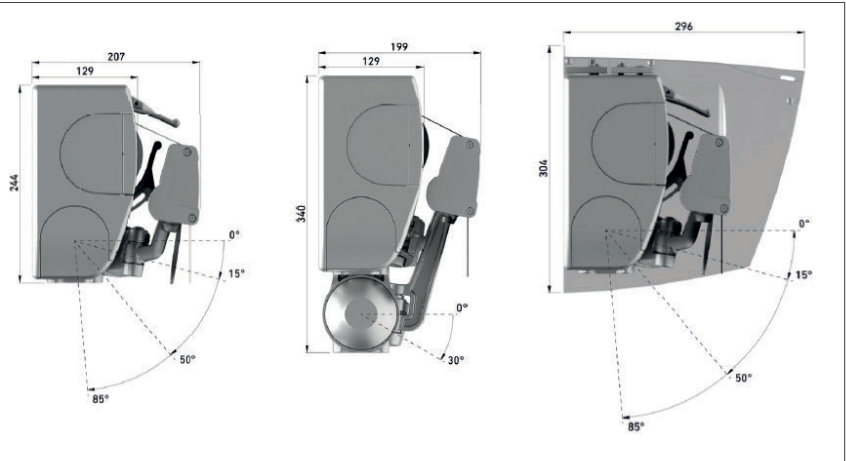
dimensiones generales
