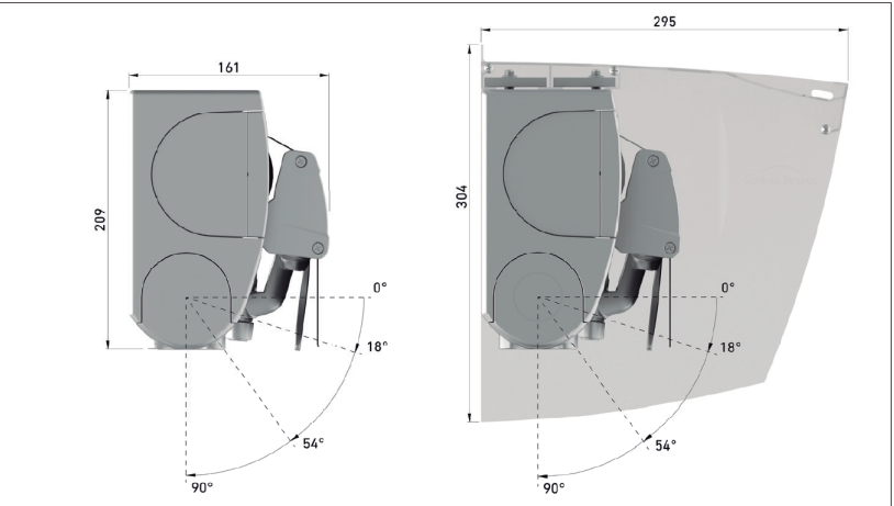
dimensiones generales
